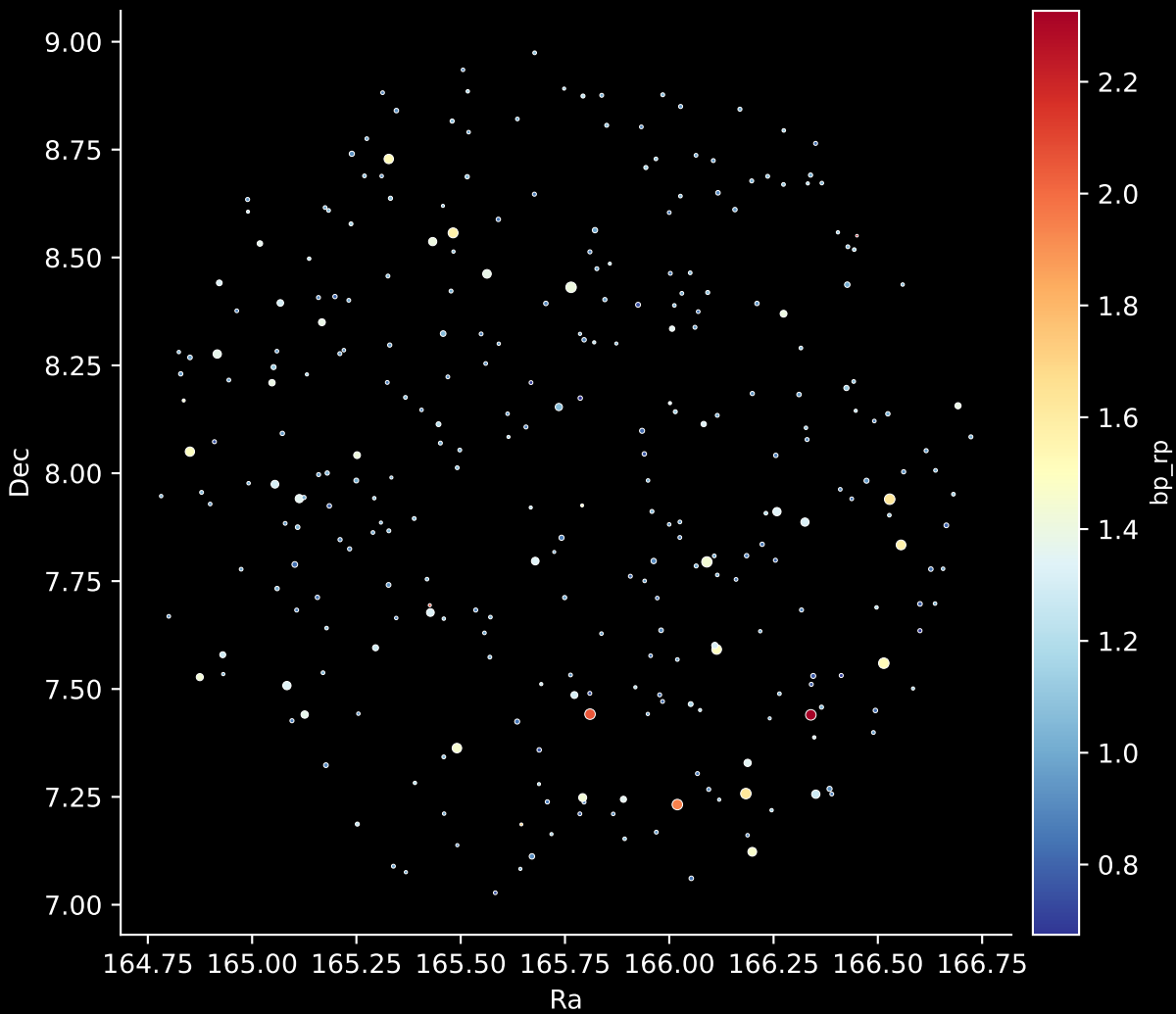
GALAH DR4 Field: [1173] Stars: 303
