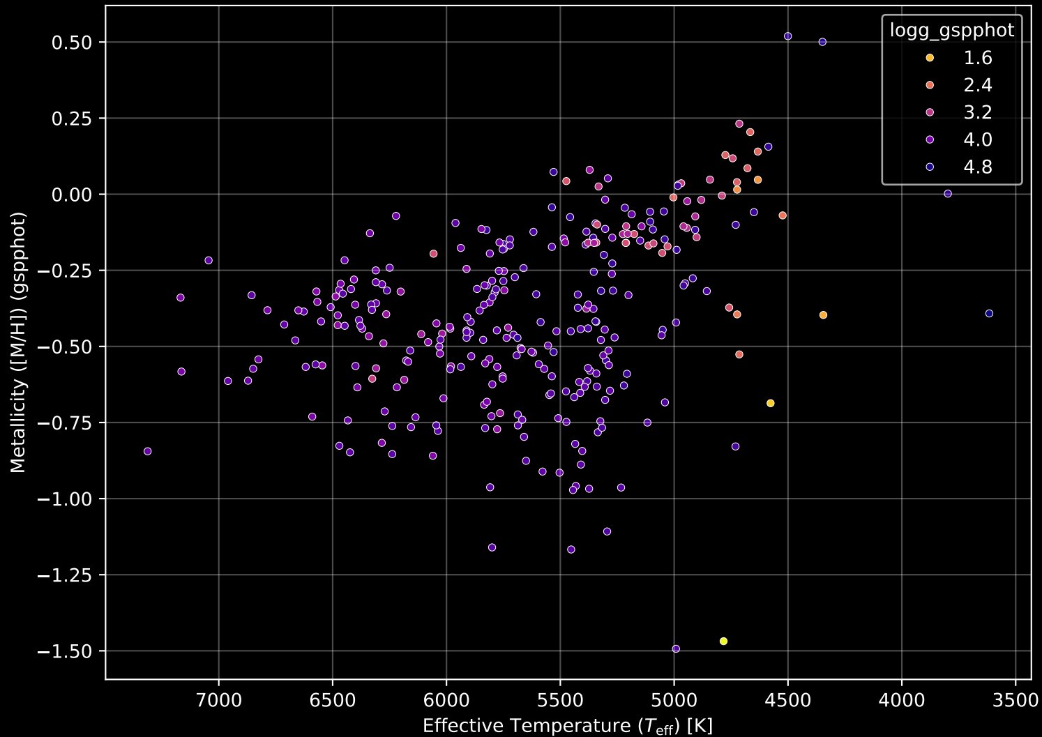
GALAH DR4 Field: [1173] Stellar Population Parameters (n= 303)
