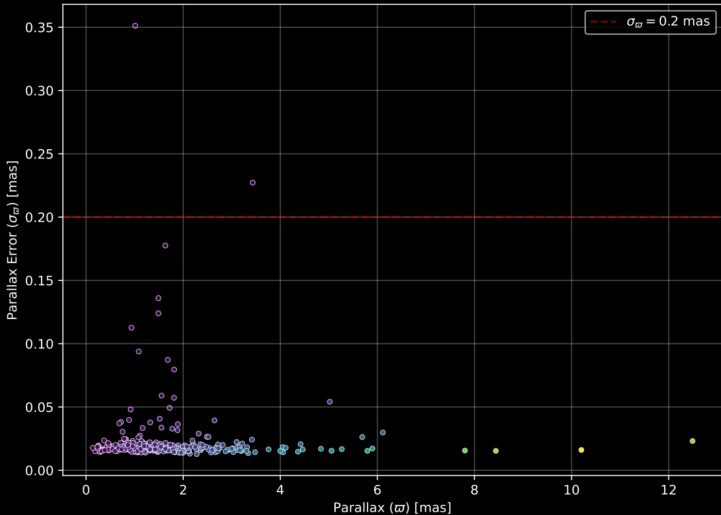
GALAH DR4 Field: [1173] Parallax Quality (n= 303)
