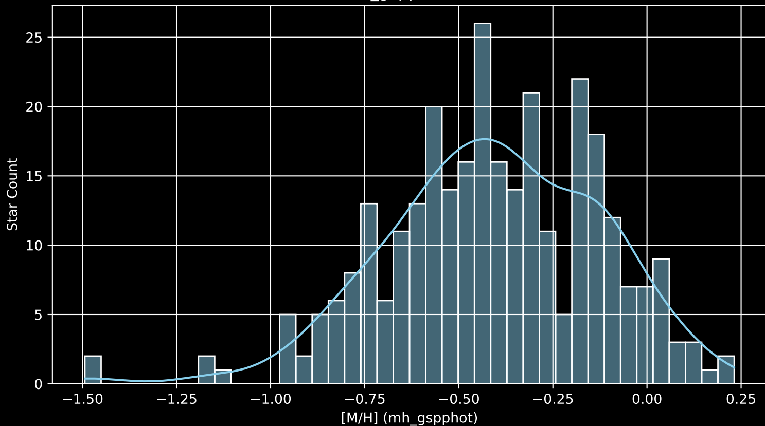
GALAH DR4 Field: [1173] [M/H] (mh_gspphot) (n= 301)
